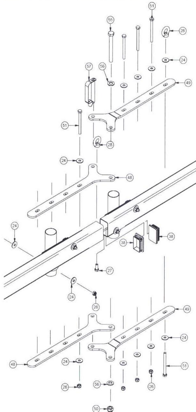
Détail M
