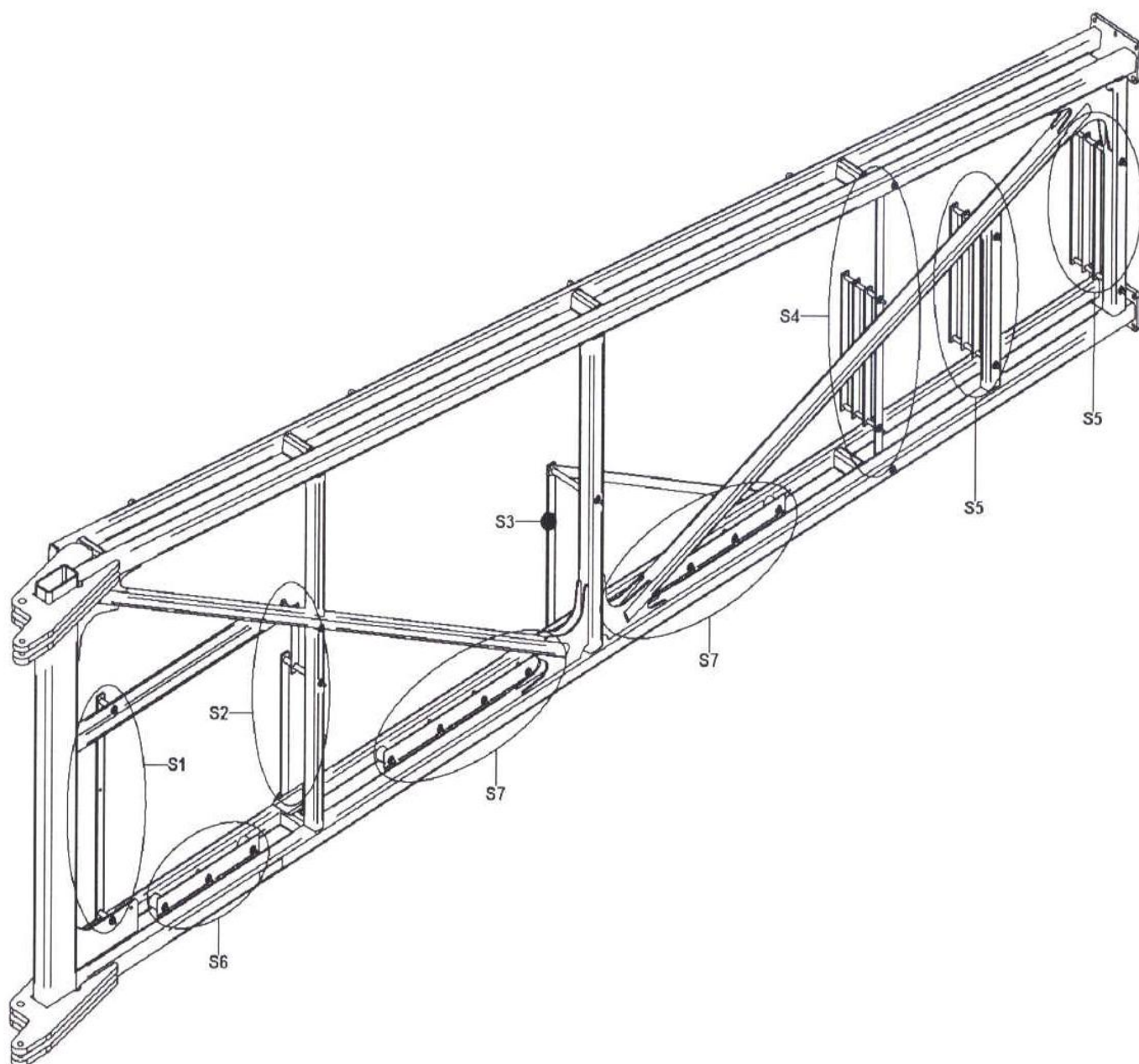
Figure E : Support de tuyau de la face interne du bras
