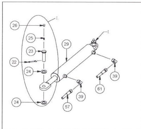
Détails G
