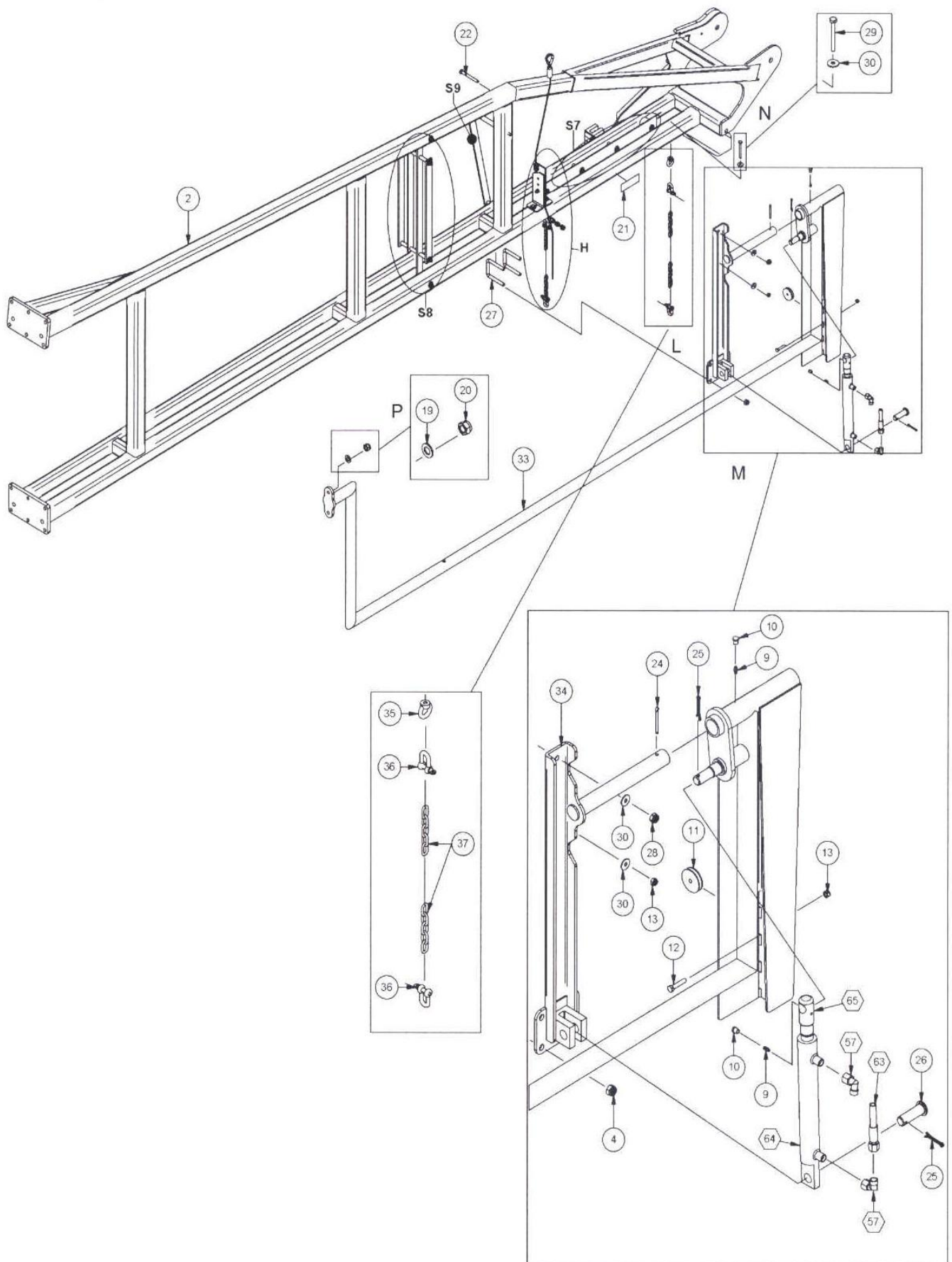
Figure D : Bras externe
