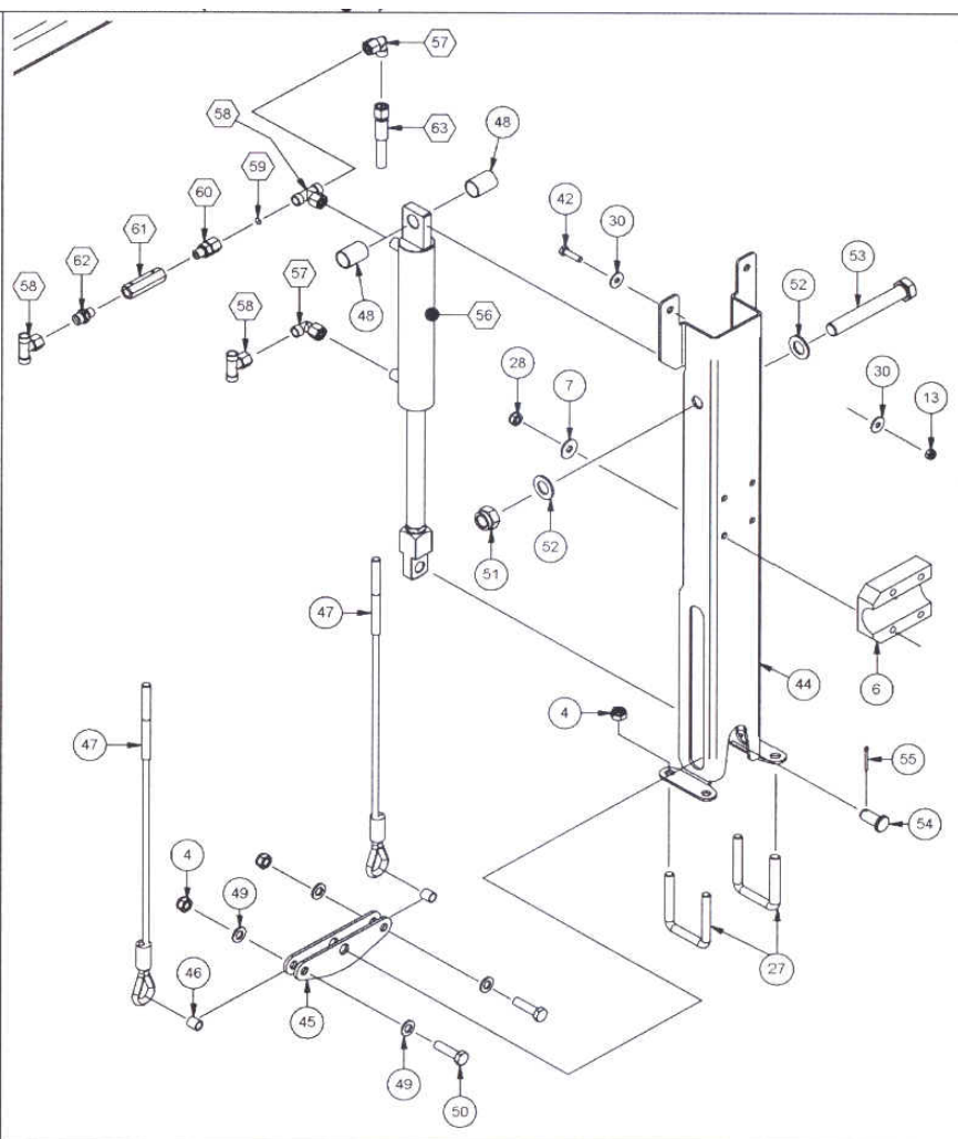
Détails K (dans figure C)
