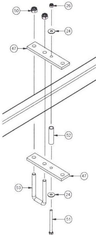
Détail E
