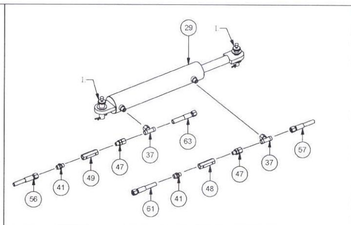
Détails H
