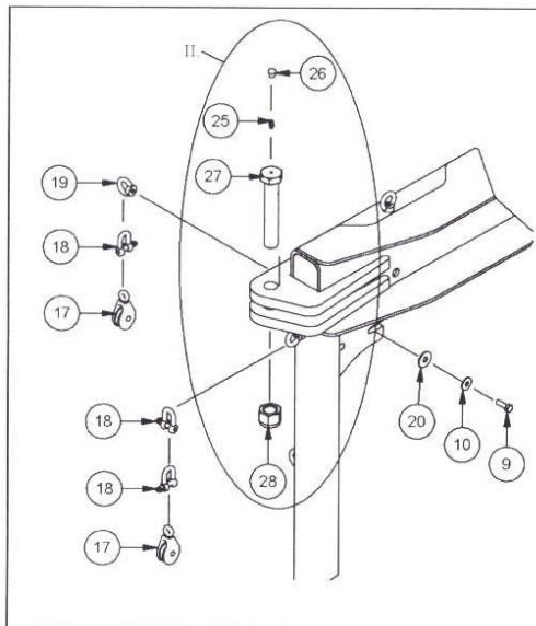
Détails E
