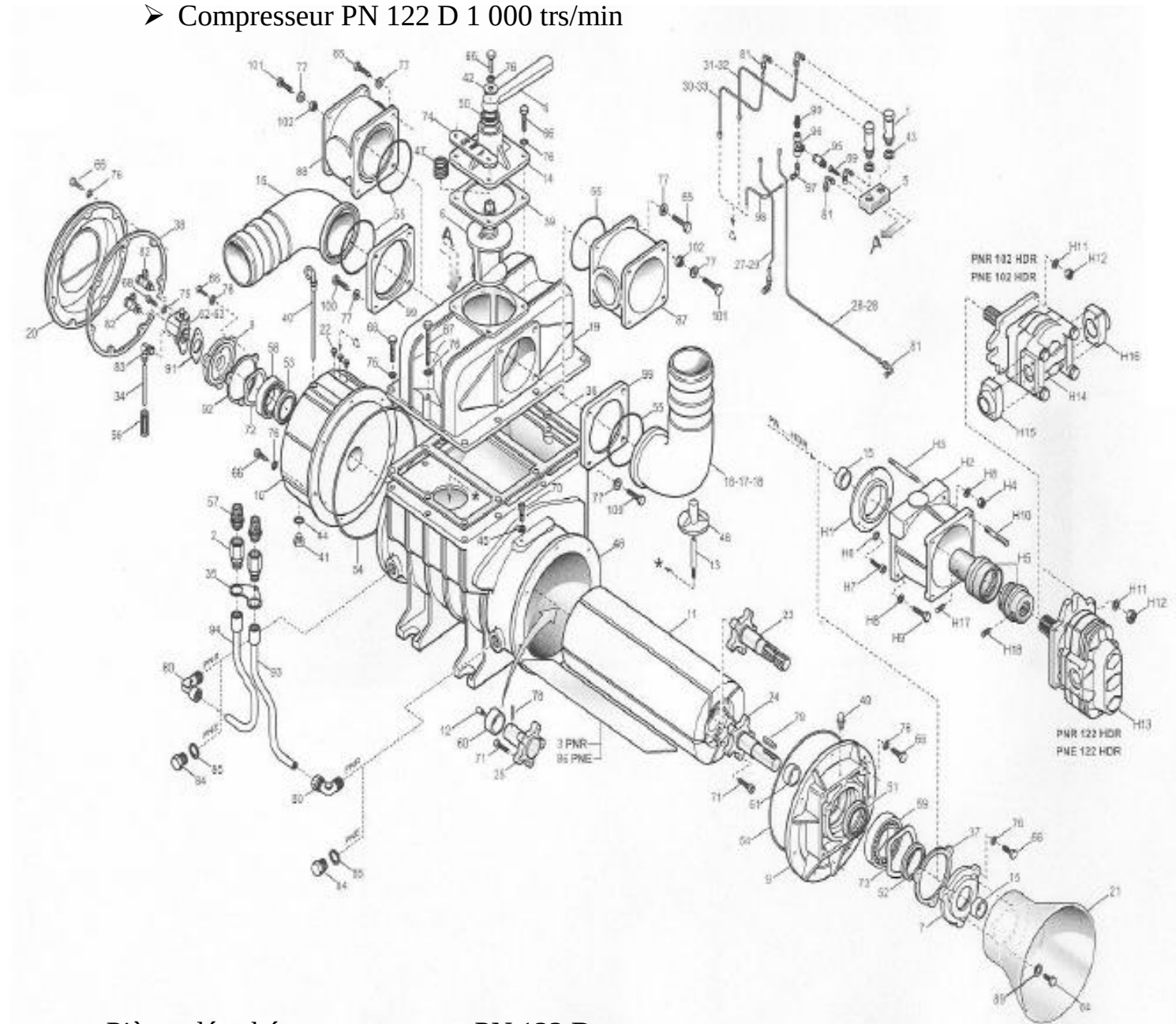
Pièces détachées compresseur PN 122 D
