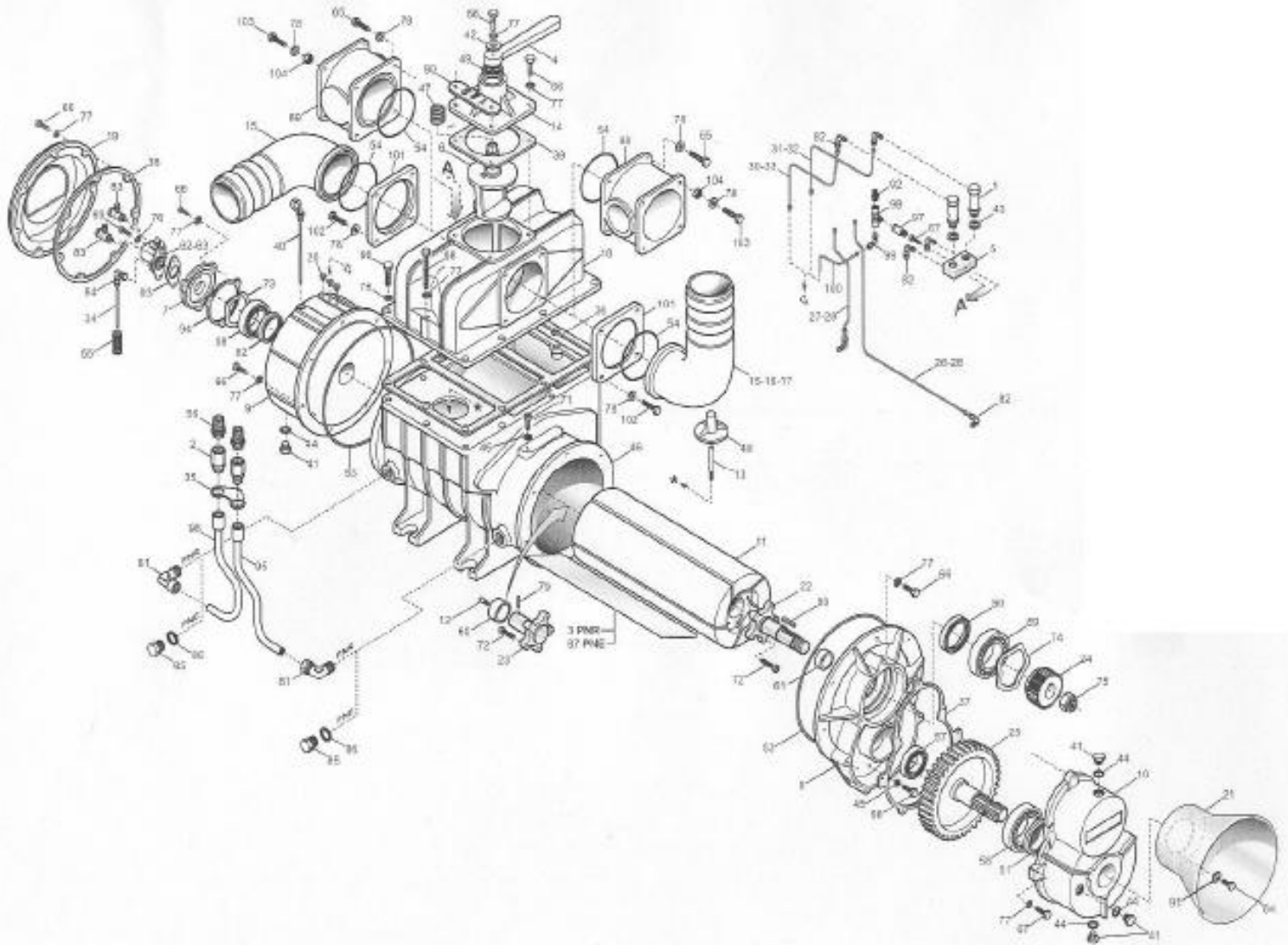
Pièces détachées compresseur PN 122
