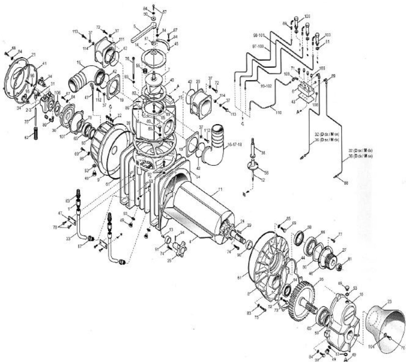
Pièces détachées compresseur 142 M
