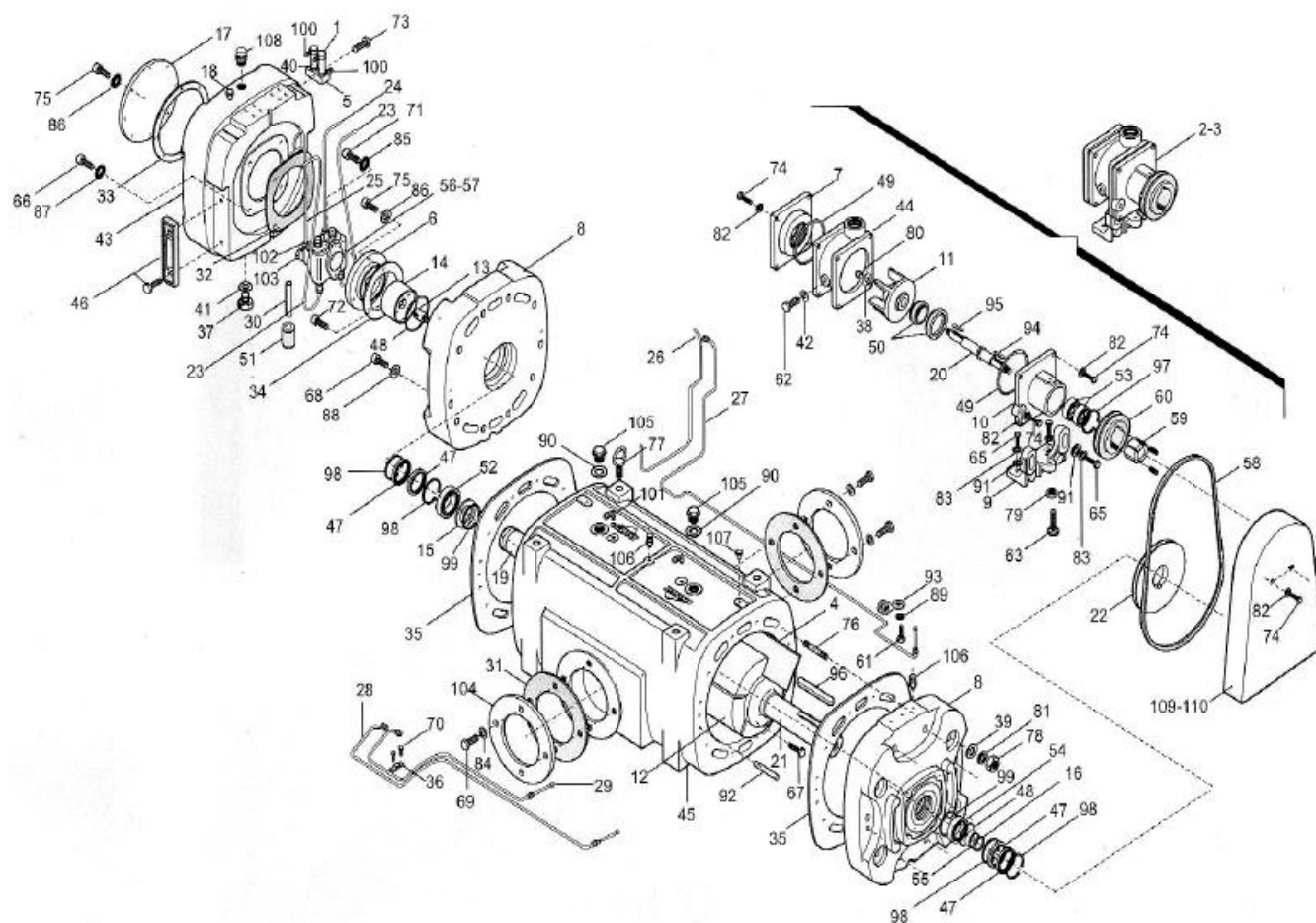
Pièces détachées compresseur PR 150 D
