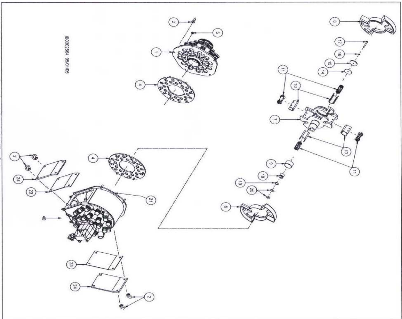
Schéma 1 : Vue éclatée des pièces d'usure de l'ExaCut
